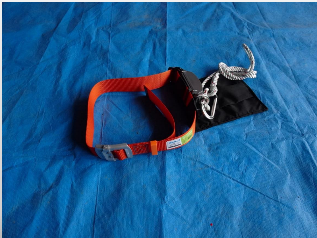
墜落制止用器具
