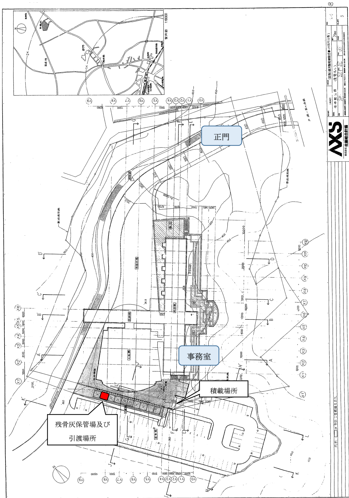
火葬場配置図
