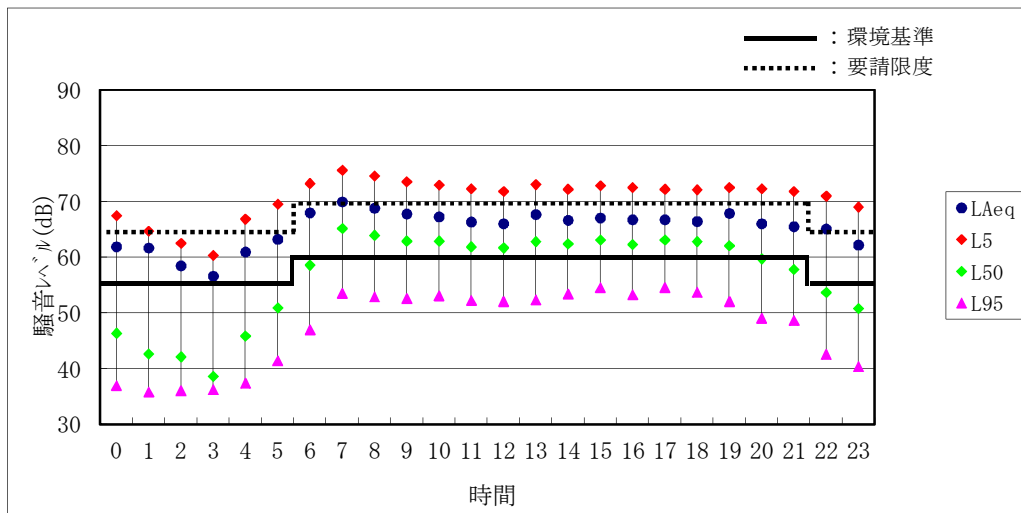
騒音レベルの時間変化
